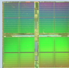
Elpida 68mm 2
