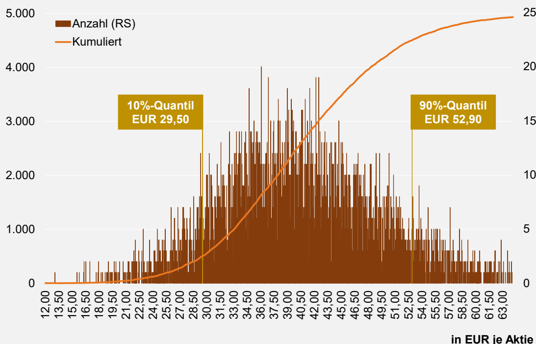
ABBILDUNG 1: MONTE-CARLO-SIMULATION (5.000 SIMULATIONEN)
