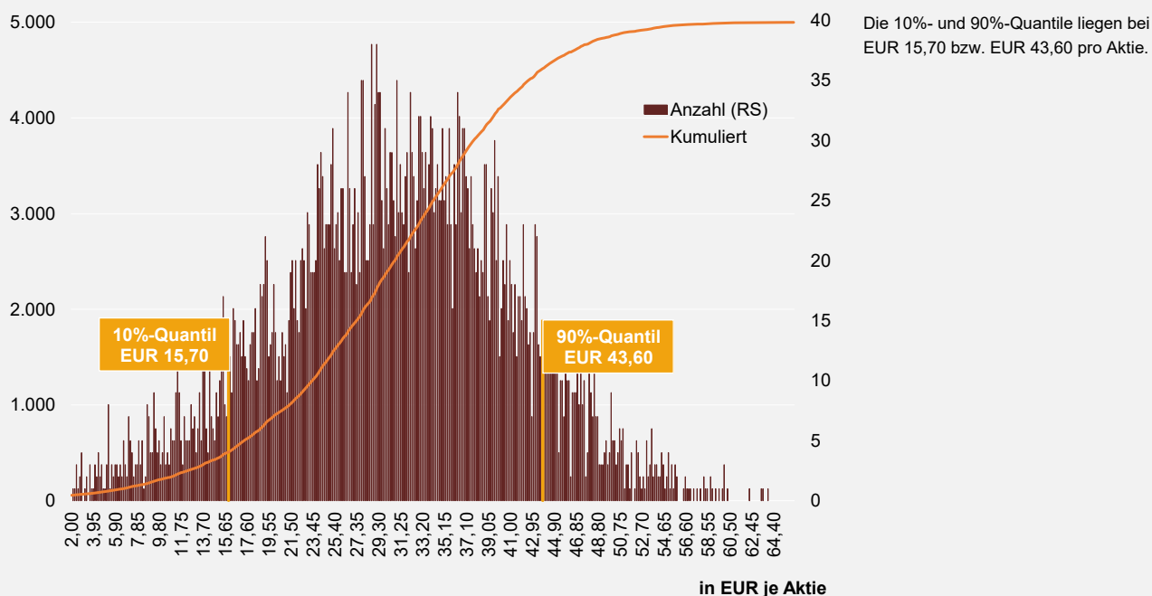
ABBILDUNG 1: MONTE-CARLO-SIMULATION
