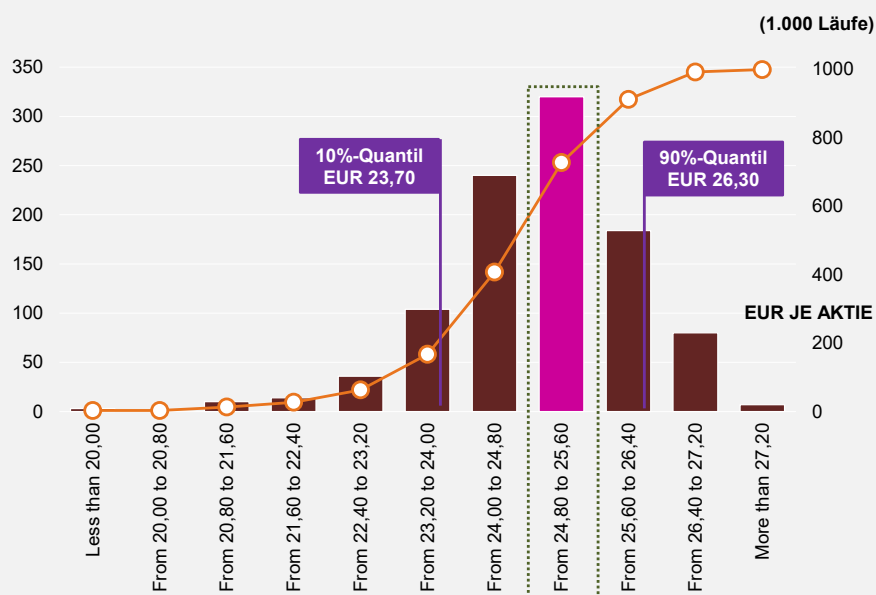
ABBILDUNG 2: MONTE-CARLO-SIMULATION
