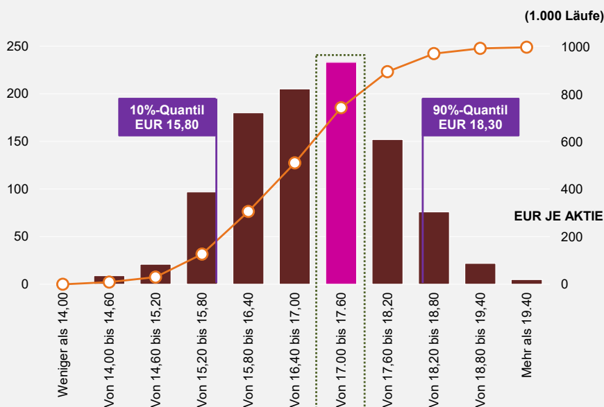
ABBILDUNG 1: MONTE-CARLO-SIMULATION
