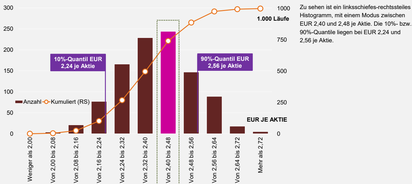
ABBILDUNG 1: MONTE-CARLO-SIMULATION
