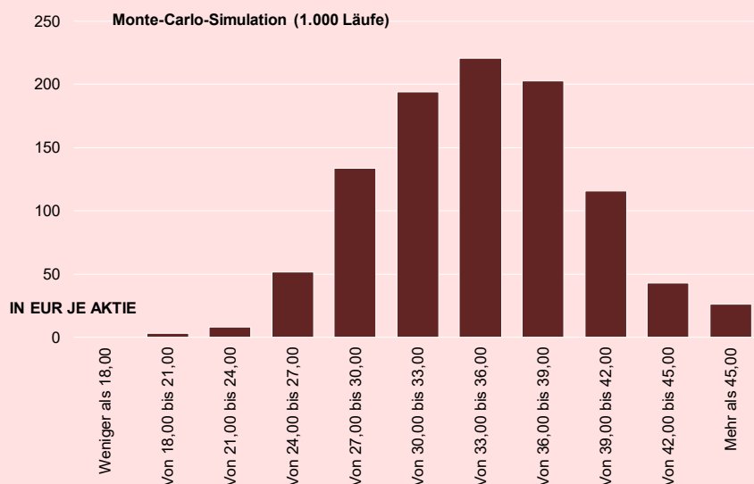
ABBILDUNG 1: ERWEITERTE SZENARIOANALYSE
