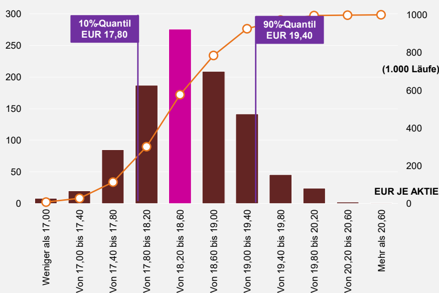
ABBILDUNG 1: MONTE CARLO-SIMULATION
