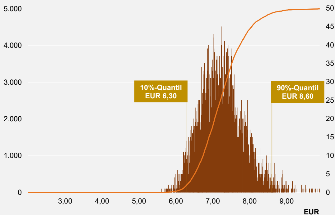
ABBILDUNG 1: MONTE-CARLO-SIMULATION (5.000 SIMULATIONEN)
