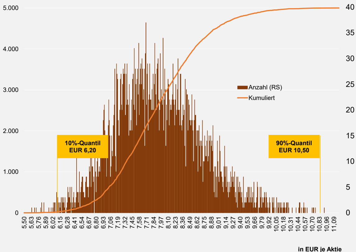
ABBILDUNG 1: MONTE-CARLO-SIMULATION (5.000 SIMULATIONEN)
