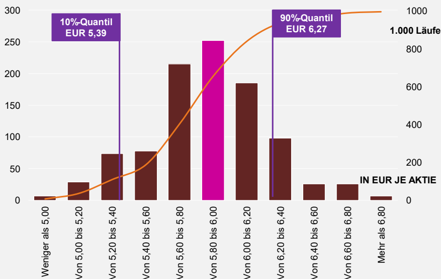
ABBILDUNG 3: MONTE CARLO-SIMULATION
