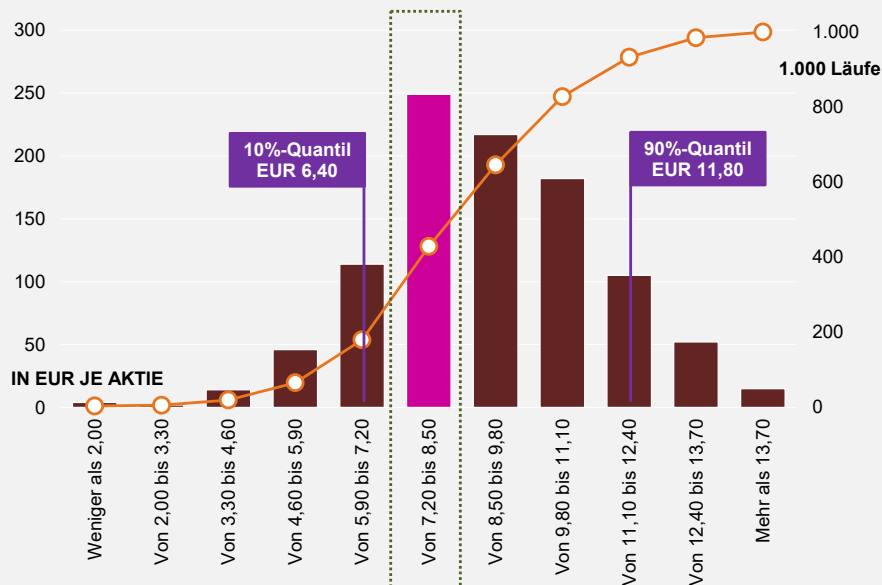
ABBILDUNG 1: MONTE CARLO-SIMULATION
